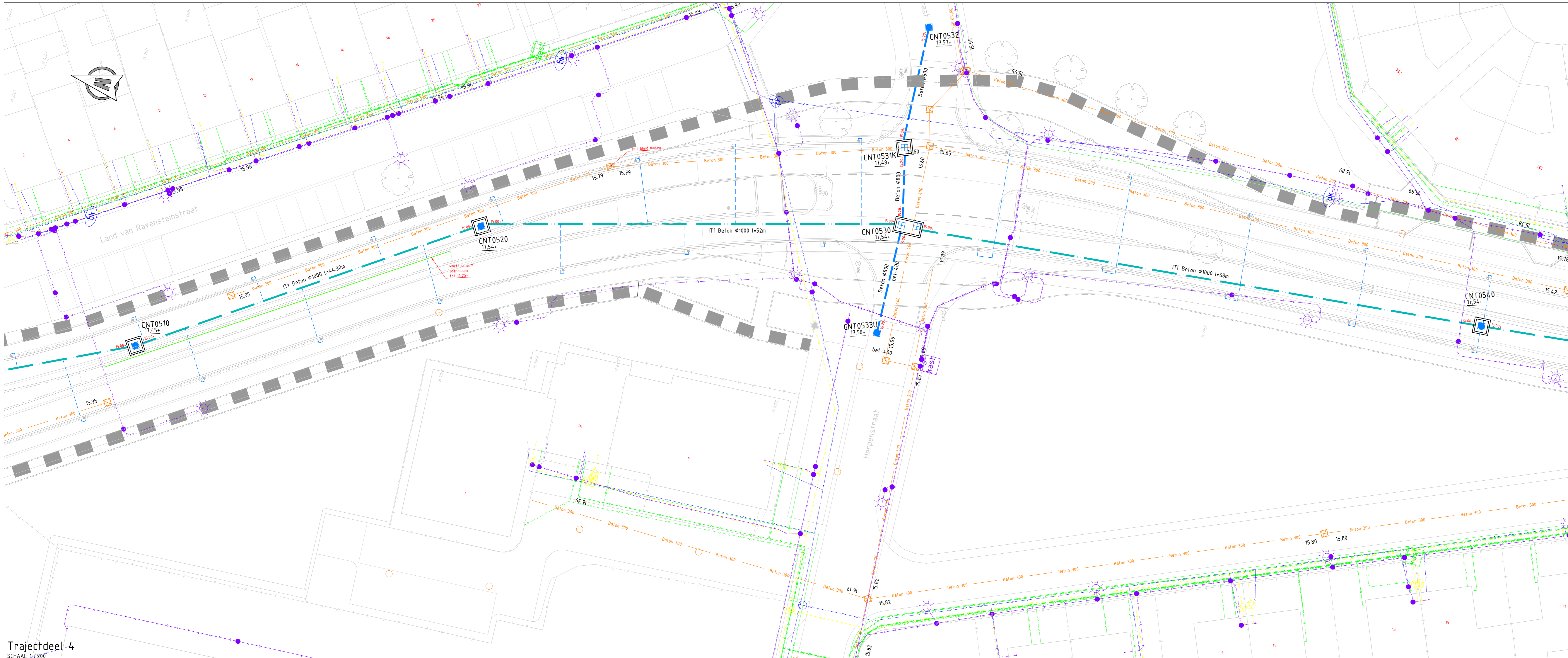
Trajectdeel 3 SCHAAL 1:200
