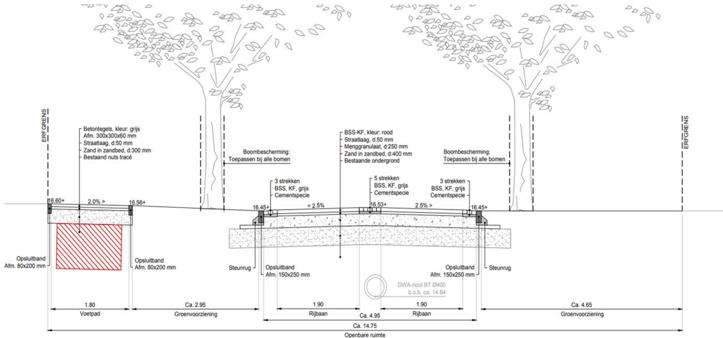
Dwarsprofiel A - A
