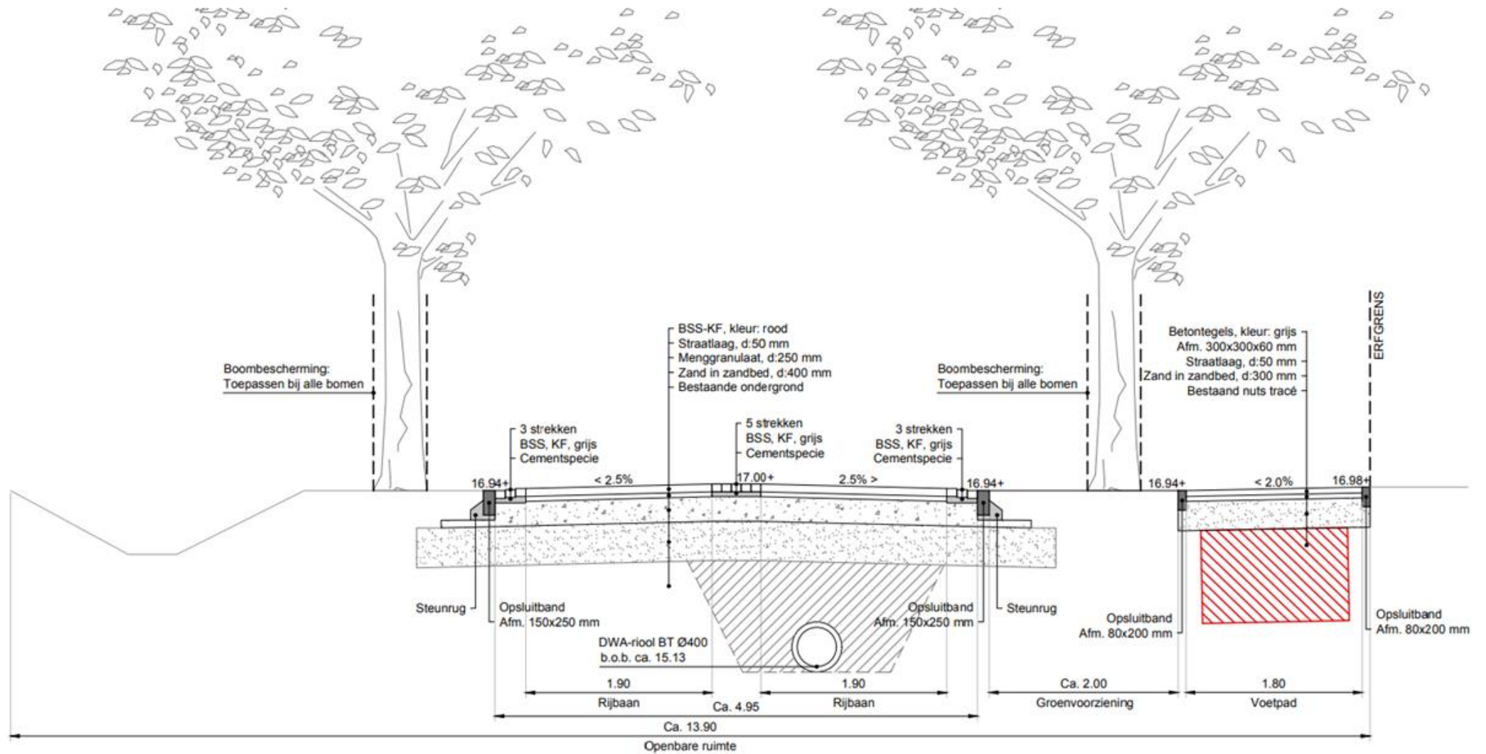
Dwarsprofiel C - C
