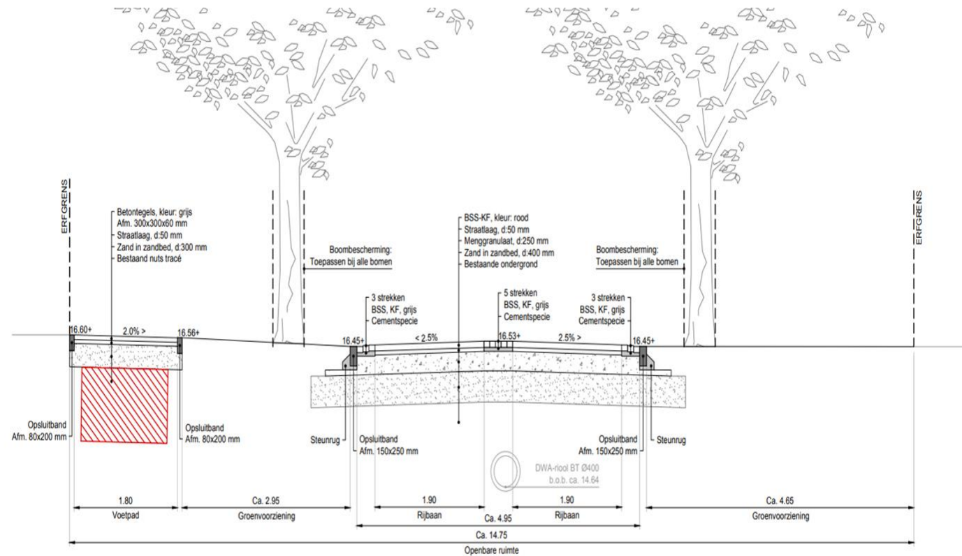
Dwarsprofiel A - A
