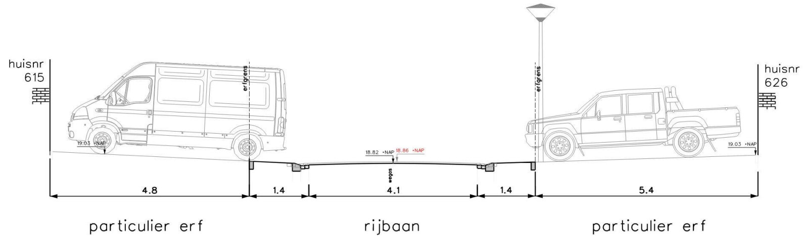
Doorsnede B - B Nieuwe situatie Schaal 1:50
