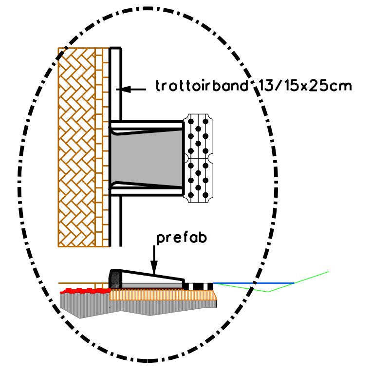
regenwater uitstroomvoorziening principe detail schaal 1:50
