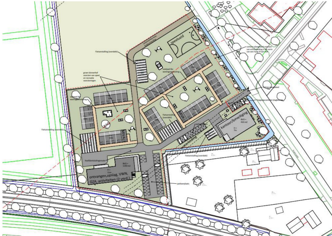
Afbeelding 3.1 Toekomstige indeling tijdelijke opvanglocatie Boekelsedijk Uden
