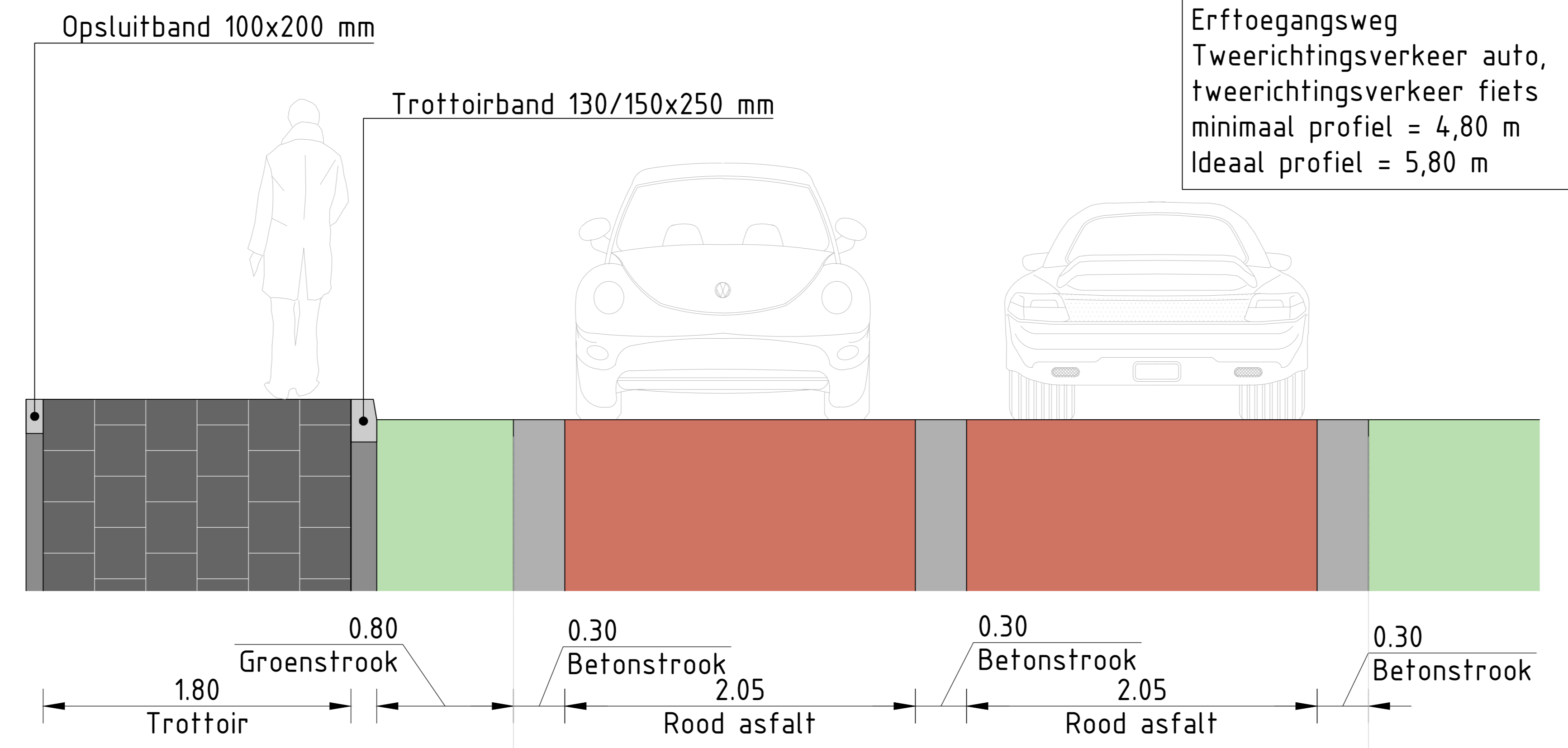
Dwarsprofiel B-B Schaal 1:20
